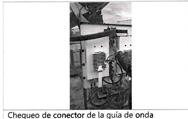
Chequeo de conector de la guía de onda
