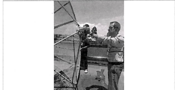
Aplicación de líquido anticorrosivo en los tornillos
