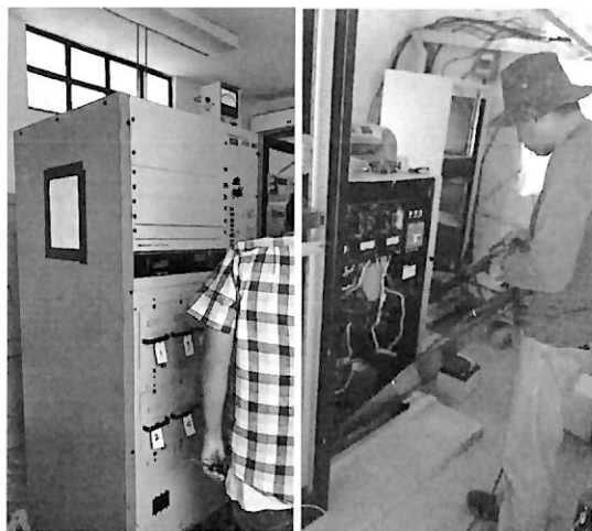
Limpieza con aspiradora del transmisor y regulador de voltaje
