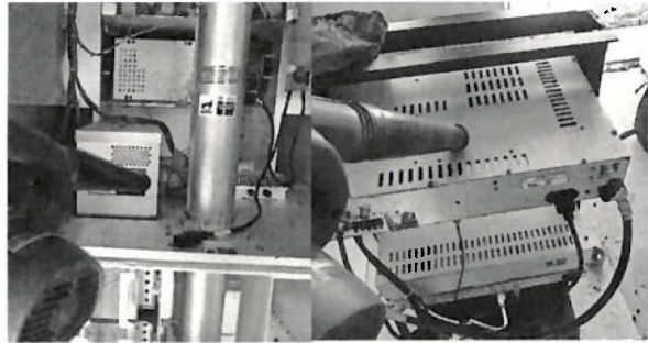
Limpieza con aspiradora del transmisor, enlace estudio-planta y monitores de modulación y estereofonía
