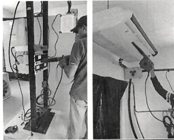
Limpieza y ajuste de equipos de transmisión y monitoreo, y del sistema de enfriamiento (clima)
